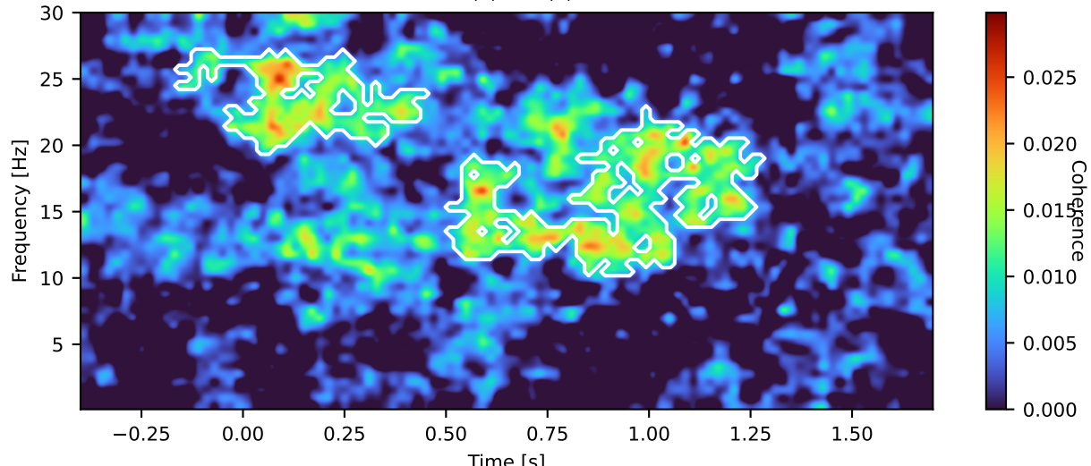
8B (0) - PE (3)
